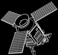
sentinel-5p
